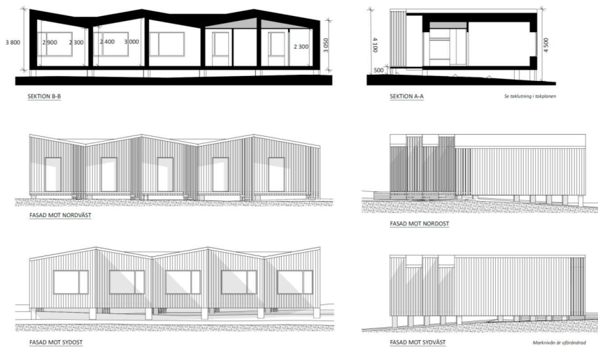
Bild 28 Fasadritningar av byggnaden som redan har fått bygglov i planområdet. Varje rum är ungefär 20 m 2 . Fasadritningar i bygglovsärendet innebär avvikelse av sex sektioner. (Bild: Nordmark arkitekter)
