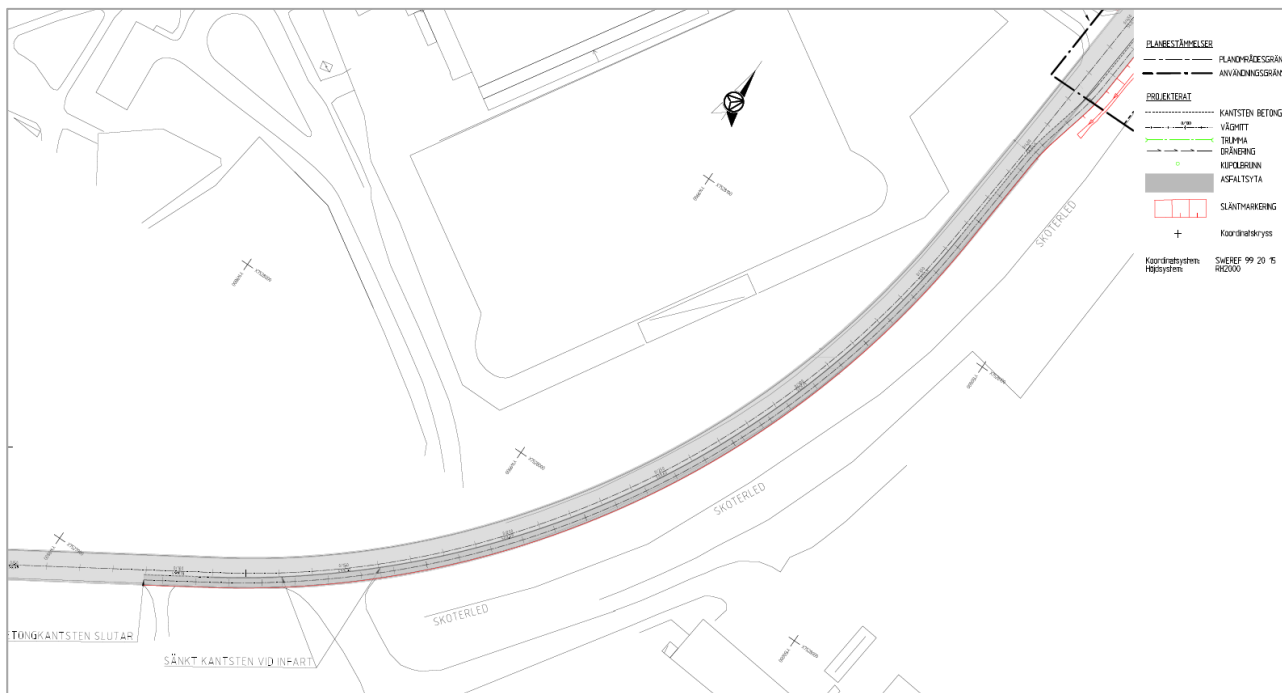
Figur 4, Principskiss på ny trafiklösning.
