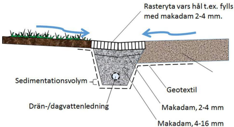
Figur 20, Illustration av krossdike med dräneringsledning i botten och makadamfyllning. Illustration från (Stockholms stad, 2023).
