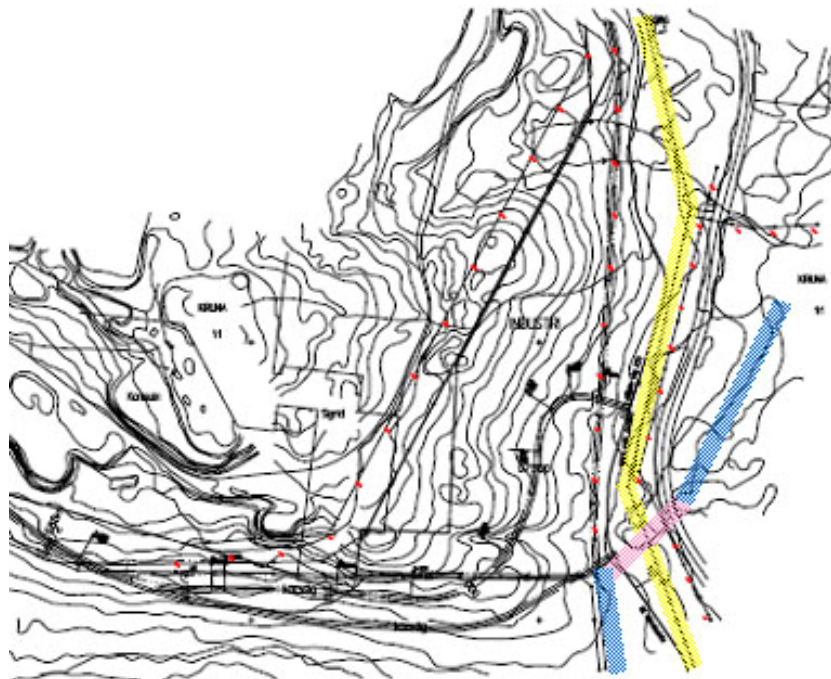
Figur 6. Översiktlig bild över de kraftledningarna som skall bibehållas samt raderas inom planområdet. De gula, rosa samt blåa linjerna kommer att behållas medan de rödprickmarkerade kraftledningarna skall raderas.
