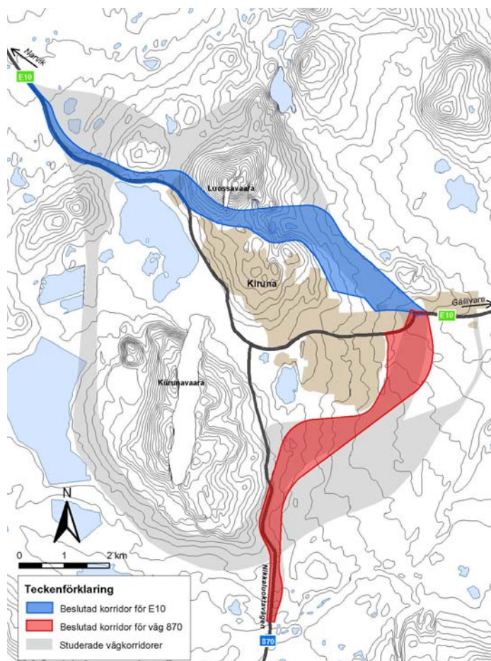
Figur 3. Beslutade vägkorridorer för väg E10 samt väg 870.
