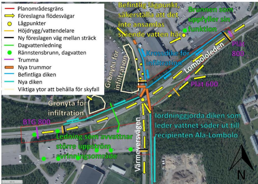
Figur 19, föreslagen systemlösning.
