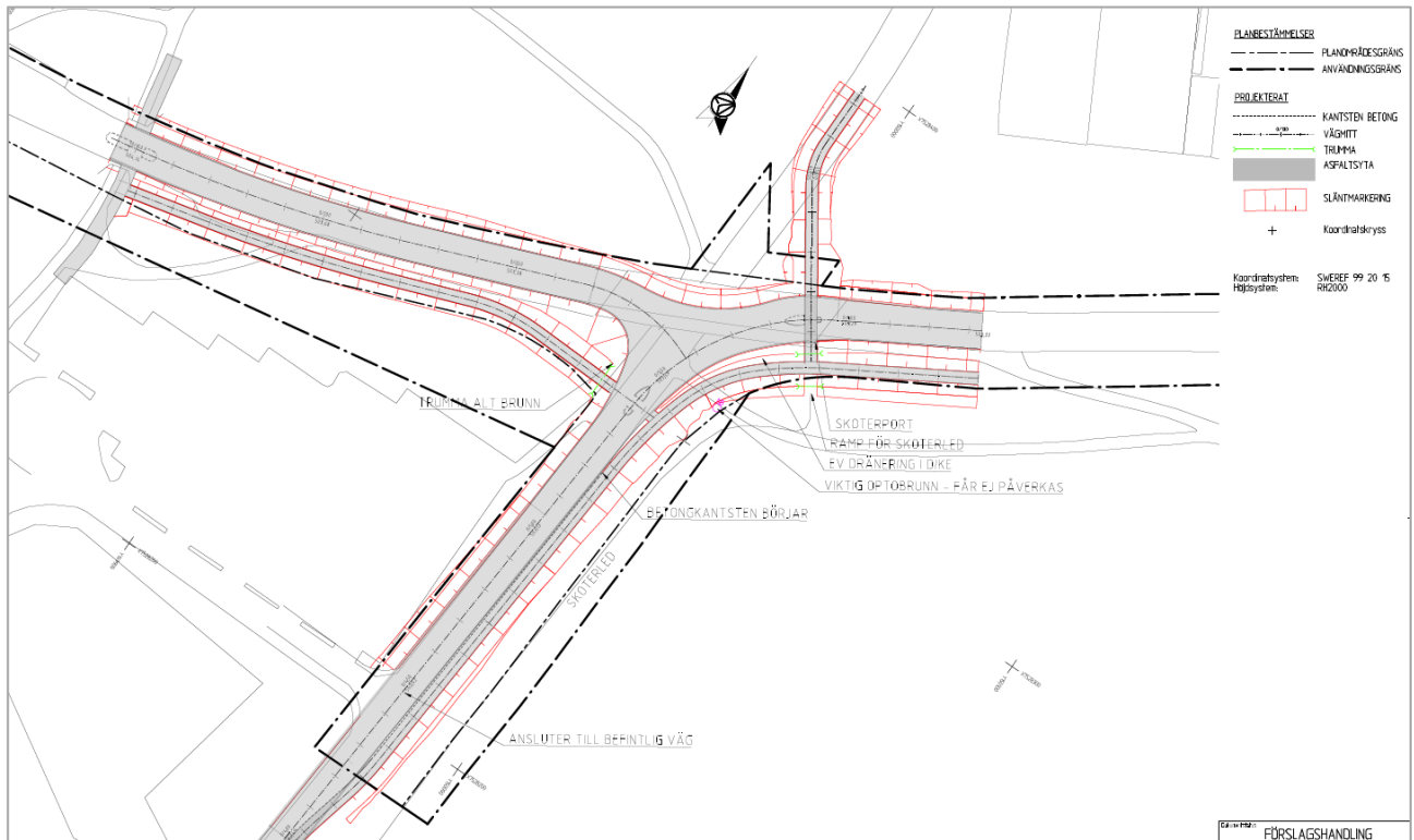
Figur 3, Principskiss på ny trafiklösning.
