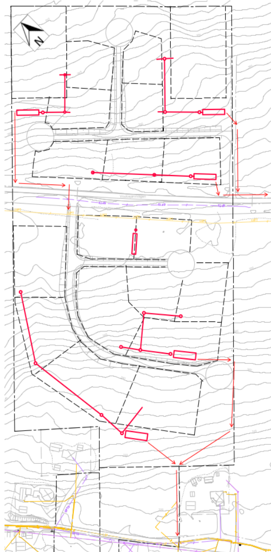
Figur 10. Föreslagen lösning med flera mindre gemensamhetsanläggningar (röda rektanglar). Föreslagen dragning av avloppsledning är visad med röda streck och släpp av rena vatten är visad med röda pilar.
